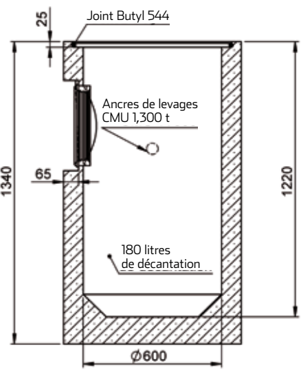
ÉLÉMENTS DE FOND Type H 1200 BM
