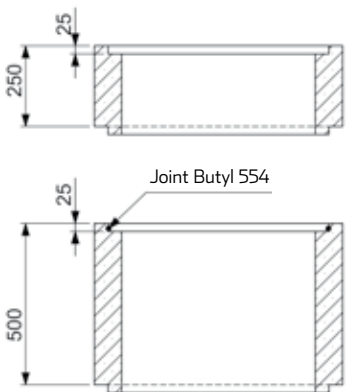
ÉLÉMENTS DROITS
