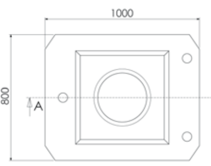
DALLE SIPHOÏDE
