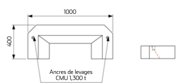
DEMI - DALLE
