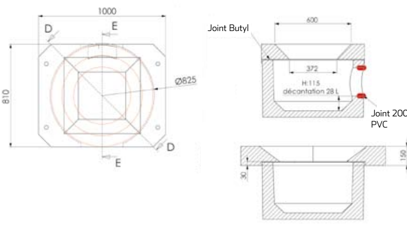
DALLE LANDES
