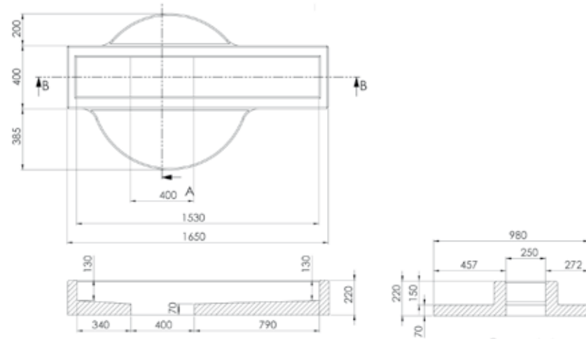
DALLE LANDES
