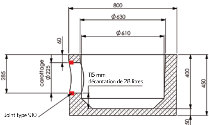
ÉLÉMENTS DE FOND Type H 450 VD
